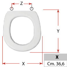
Cerniera universale cromato
